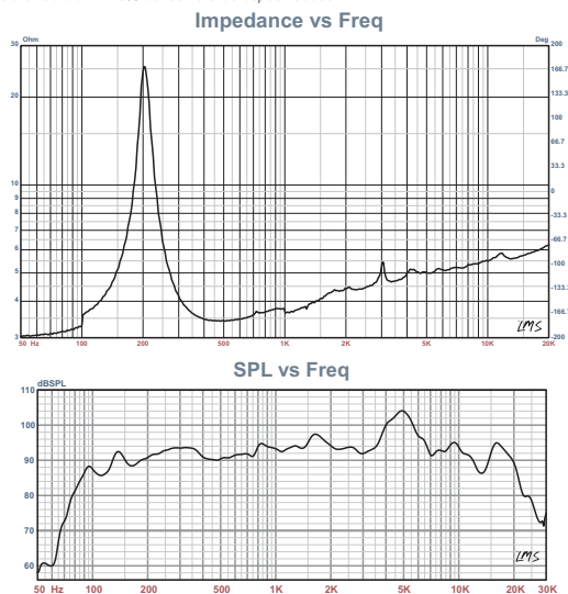
Curva de respuesta obtenida num box de 8L x 110Hz (1W x 1m).
